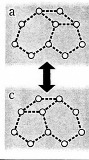
準結晶の構造の揺らぎ
